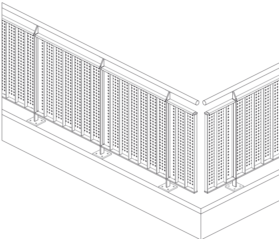
3D du barreaudage de l'extérieur
