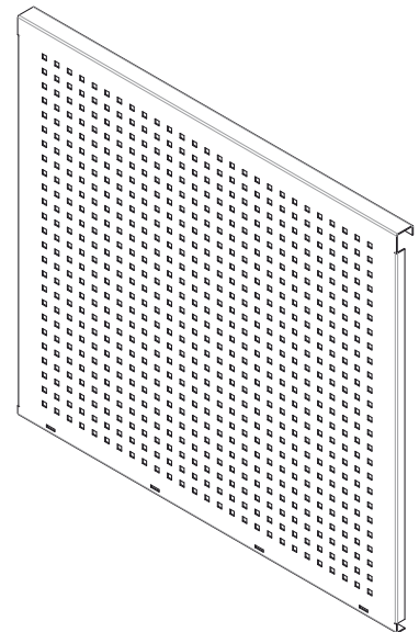
3D Ansicht Geländerblende von innen
